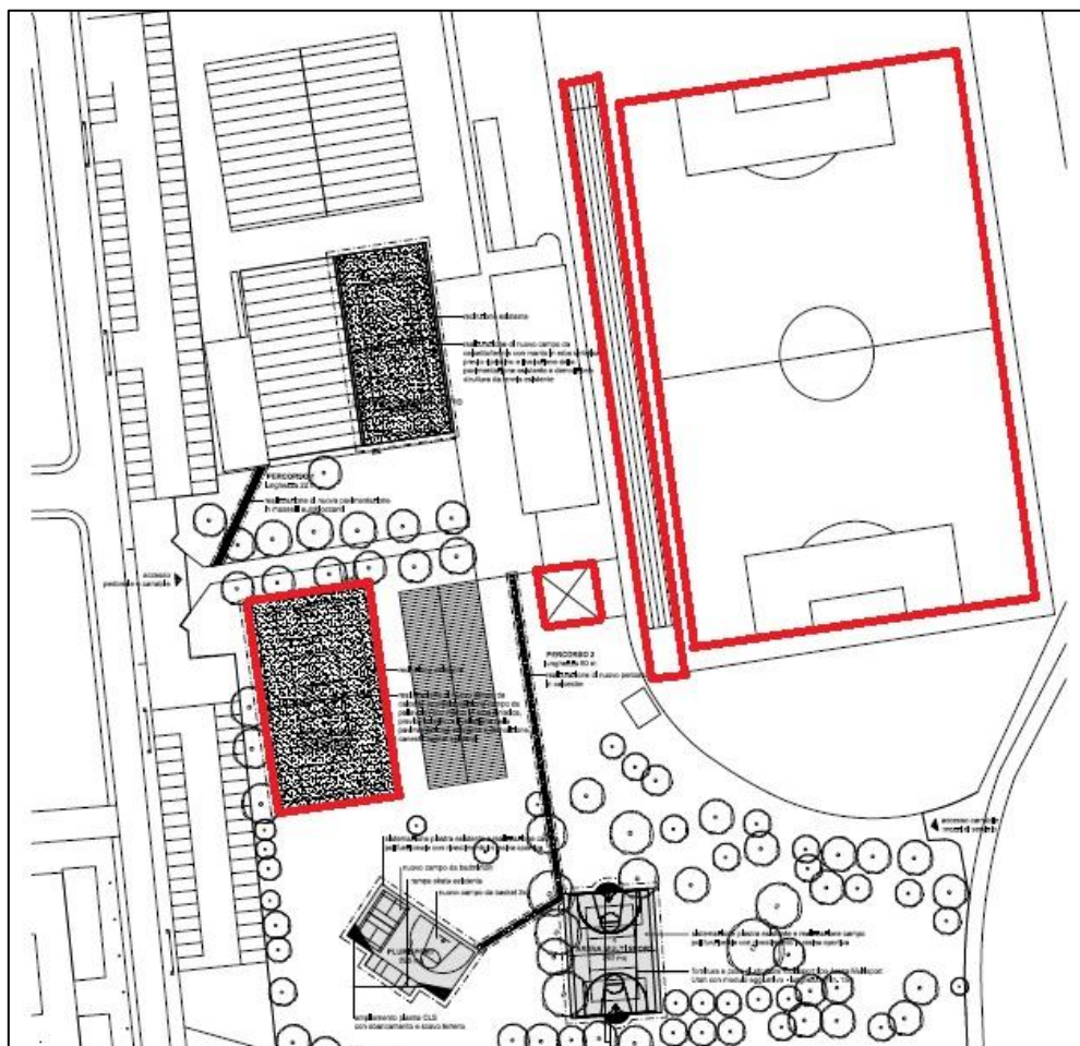
Planimetria generale.
